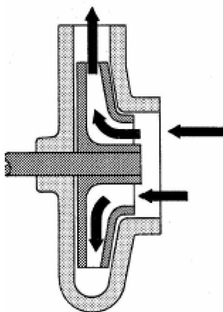
IMPELLER
